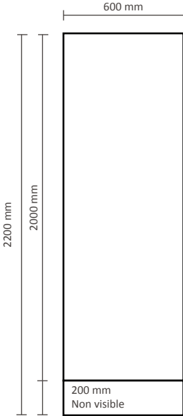
60x200cm RBCUBE060
